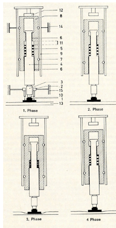
Abb. 4: „Künstlicher Sportler Stuttgart“, Prüfgerät zur Messung der Standardverformung von Sportböden (Quelle: BISp)
